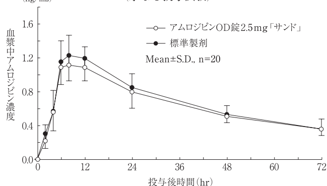
アムロジピンOD錠2.5mg「サンド」投与後の血漿中濃度推移 (水なし投与試験)
