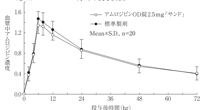
アムロジピンOD錠2.5mg「サンド」投与後の血漿中濃度推移 (水あり投与試験)
