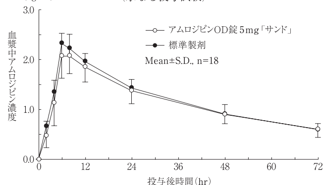
アムロジピンOD錠5mg「サンド」投与後の血漿中濃度推移 (水なし投与試験)
