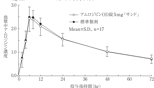
アムロジピンOD錠5mg「サンド」投与後の血漿中濃度推移 (水あり投与試験)
