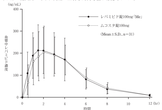
図 100mg錠投与時の血漿中レバミピド濃度推移
